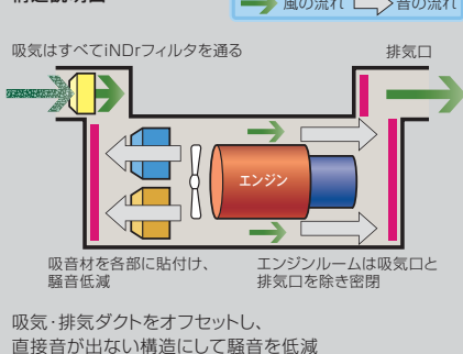
構造説明図
