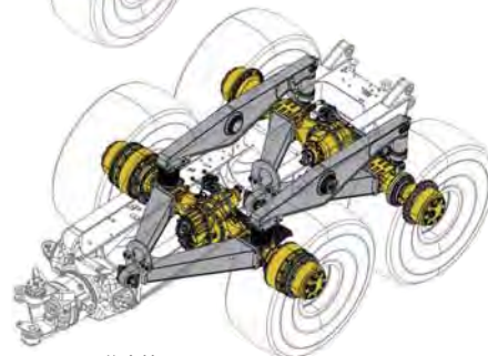
後車軸
